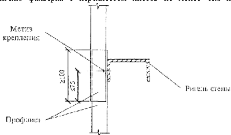
Рис. 15. Стык стеновых профлистов
