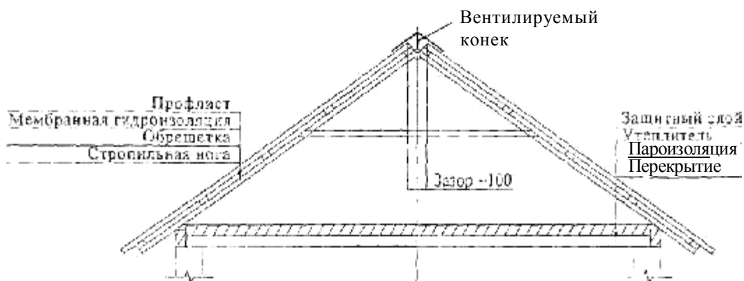
Рис. 9 Холодное чердачное помещение
