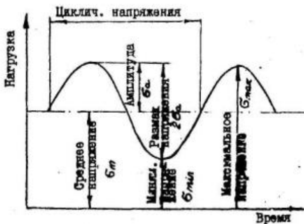
Рисунок 4 - Цикл напряжений при испытании на усталость
