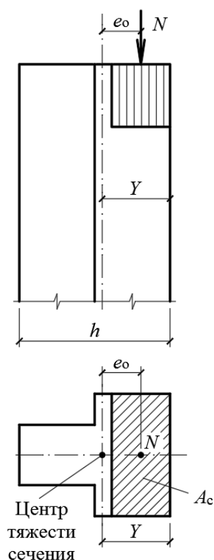
Рисунок 7.2 – Внецентренное сжатие
