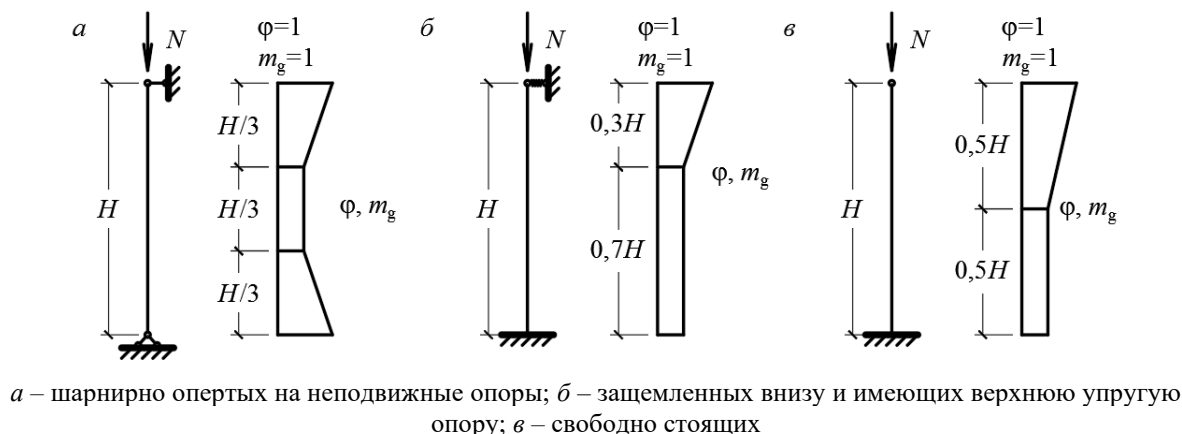
Рисунок 7.1 – Коэффициенты \varphi и m_q по высоте сжатых стен и столбов
