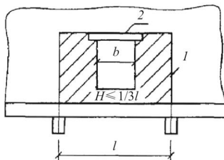
1 – нагрузка на рандбалку; 2 – железобетонная перемычка
