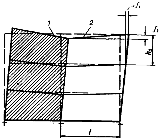
Черт. 6. Схема перекося этажных ячеек 2, примыкающих к диафрагмам жесткости 1 в зданиях со связевым каркасом (пунктиром показана исходная схема каркаса до приложения нагрузки)
