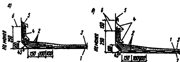
Рис 1 Примеры примыканий кровель
