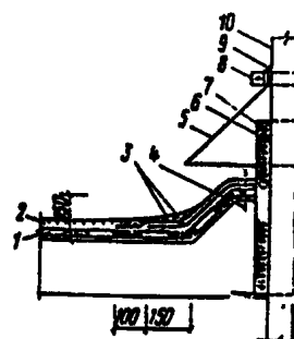
Рис 3. Пример решения пропуска труб
