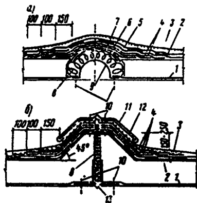
Рис 2 Примеры решений деформационных швов
