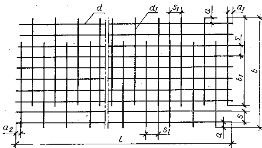
Черт.2
