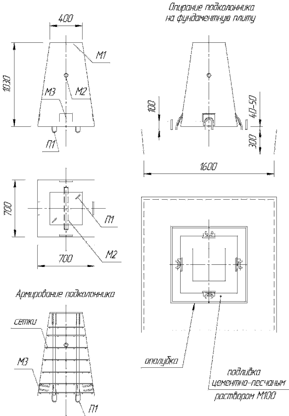
Рис. 6.3. Конструктивное решение столбчатого фундамента из сборных элементов под колонны (подколоники КНС-2 по РС1365-91 с плоским стальным торцом и фундаментной плиты ФП-16.16-35, ФП-20.20-35, ФП-20.20-35 по РС1261-93 территориального каталога типовых изделий для строительства в г. Москве)
