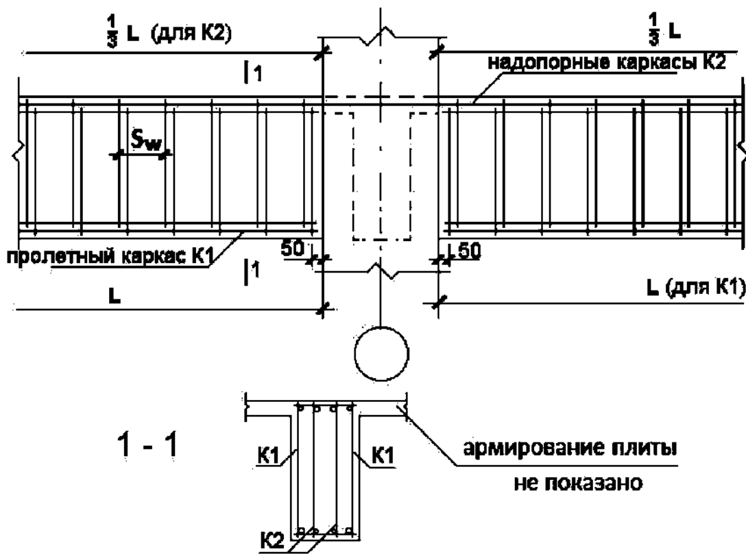
Рис. 10.4. Схема армирования контурных балок
