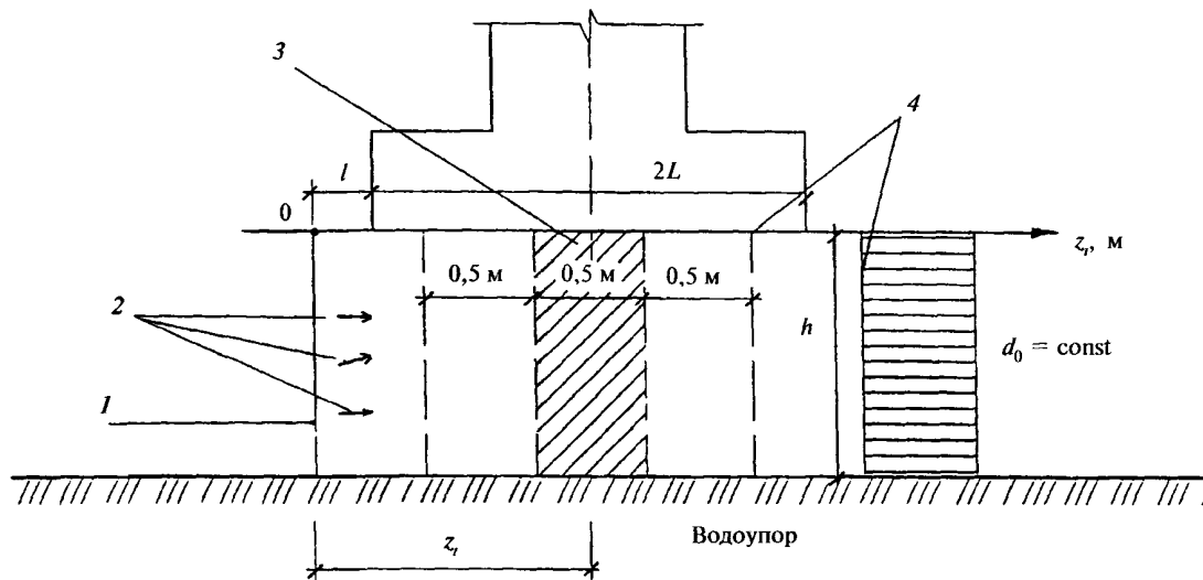
Рисунок 6.6 — Схема для расчета рассоления основания при горизонтальной фильтрации
