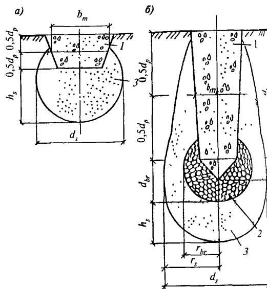
а — фундамент мелкого заложения с плоской подошвой б — удлиненный фундамент с уширенным основанием, 1 — фундамент, 2 — втрамбованный жесткий материал, 3 — уплотненная зона
