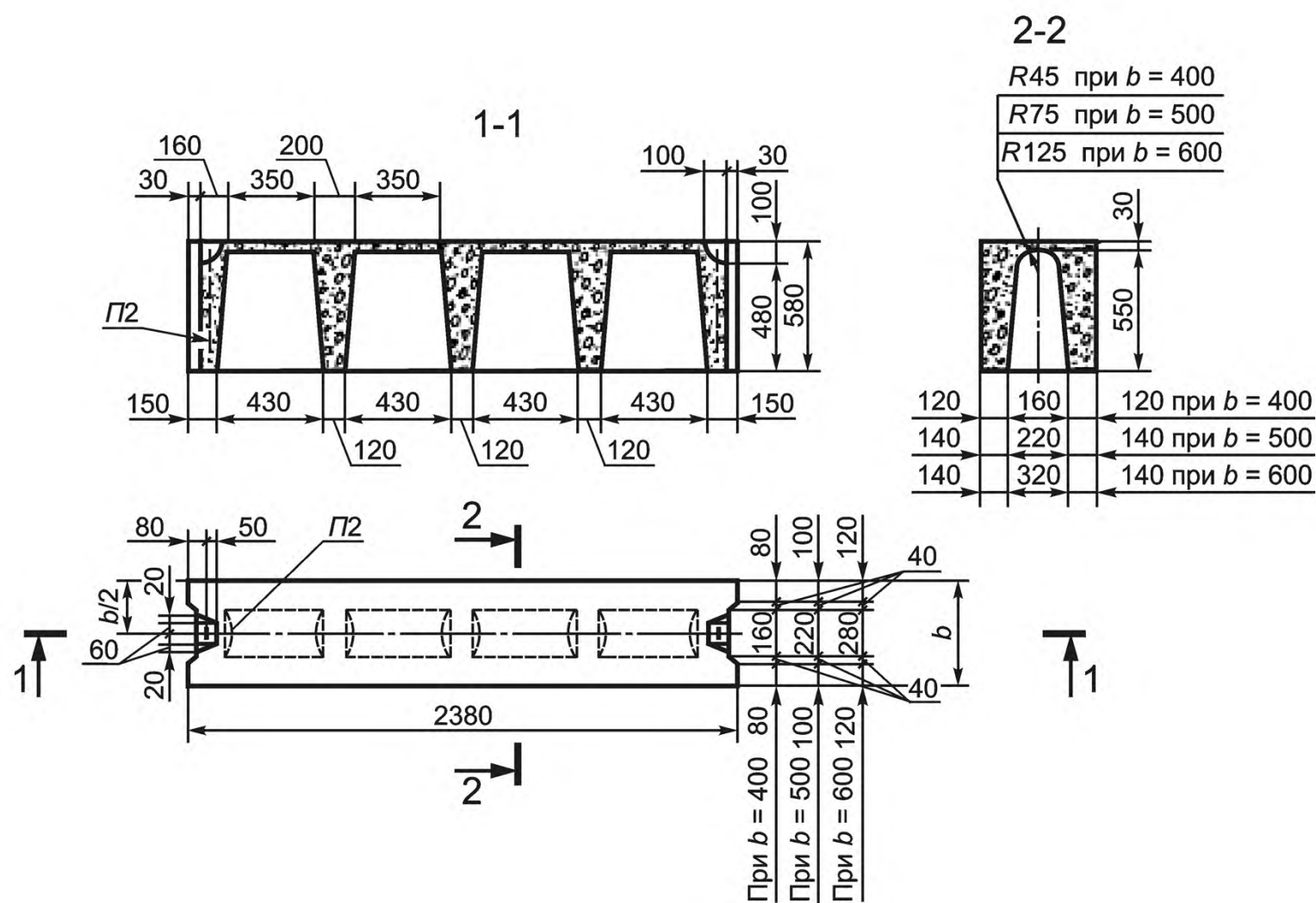
Рисунок 2 — Блоки типа ФБВ
