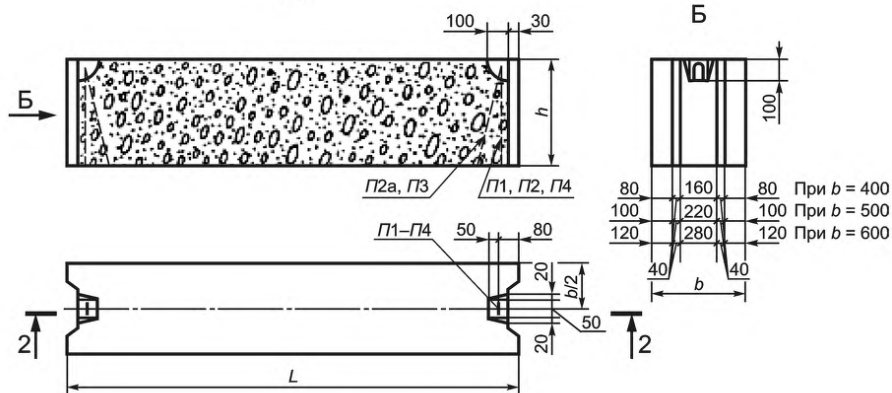
Рисунок 1 — Блоки типа ФБС
